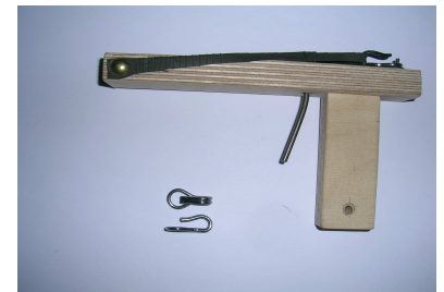
Pistola de ganxets
